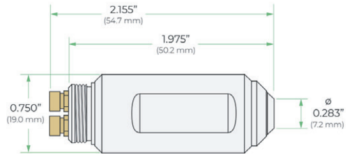
DHT-410
