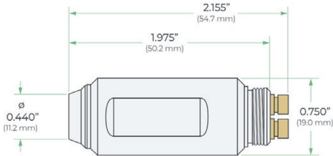
DHT-400
